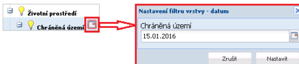
Obrázek 8 Historizace dat
