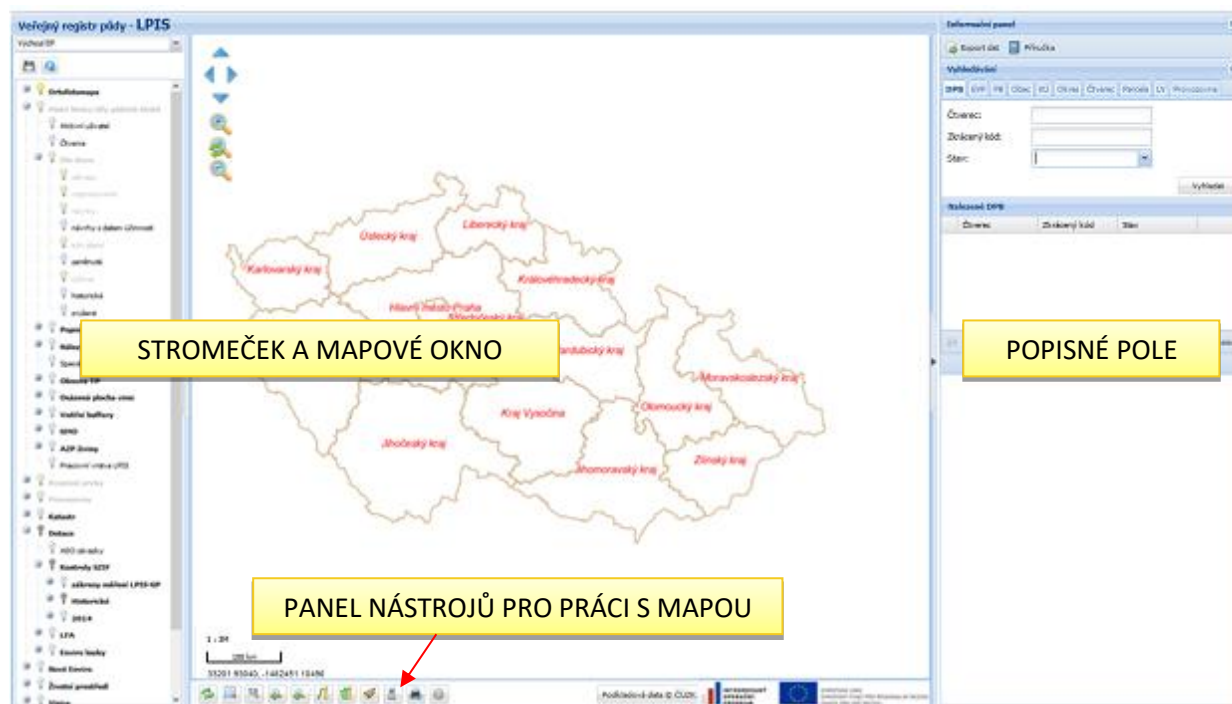
Obrázek 2 Uživatelské prostředí
