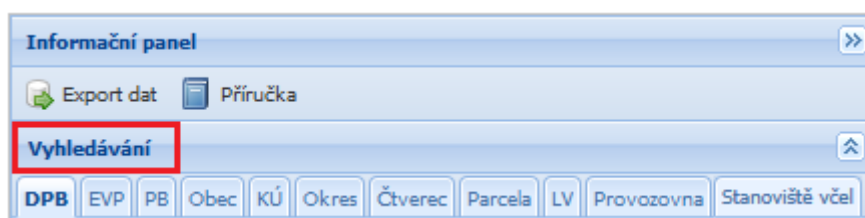
Obrázek 30 Možnosti vyhledávání
