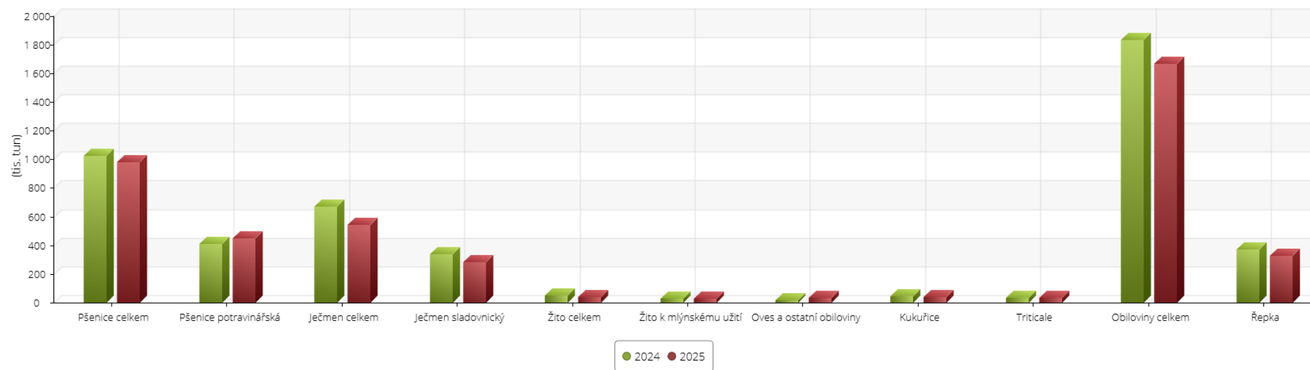
Graf - Konečná zásoba obilovin a řepky na internet (tis. tun) (3.čtvrtletí 2025/2024)
