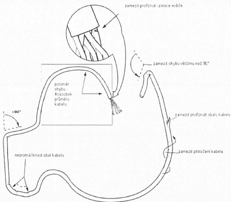
Obrázek: Dovolené a zakázané ohyby na kabelech
