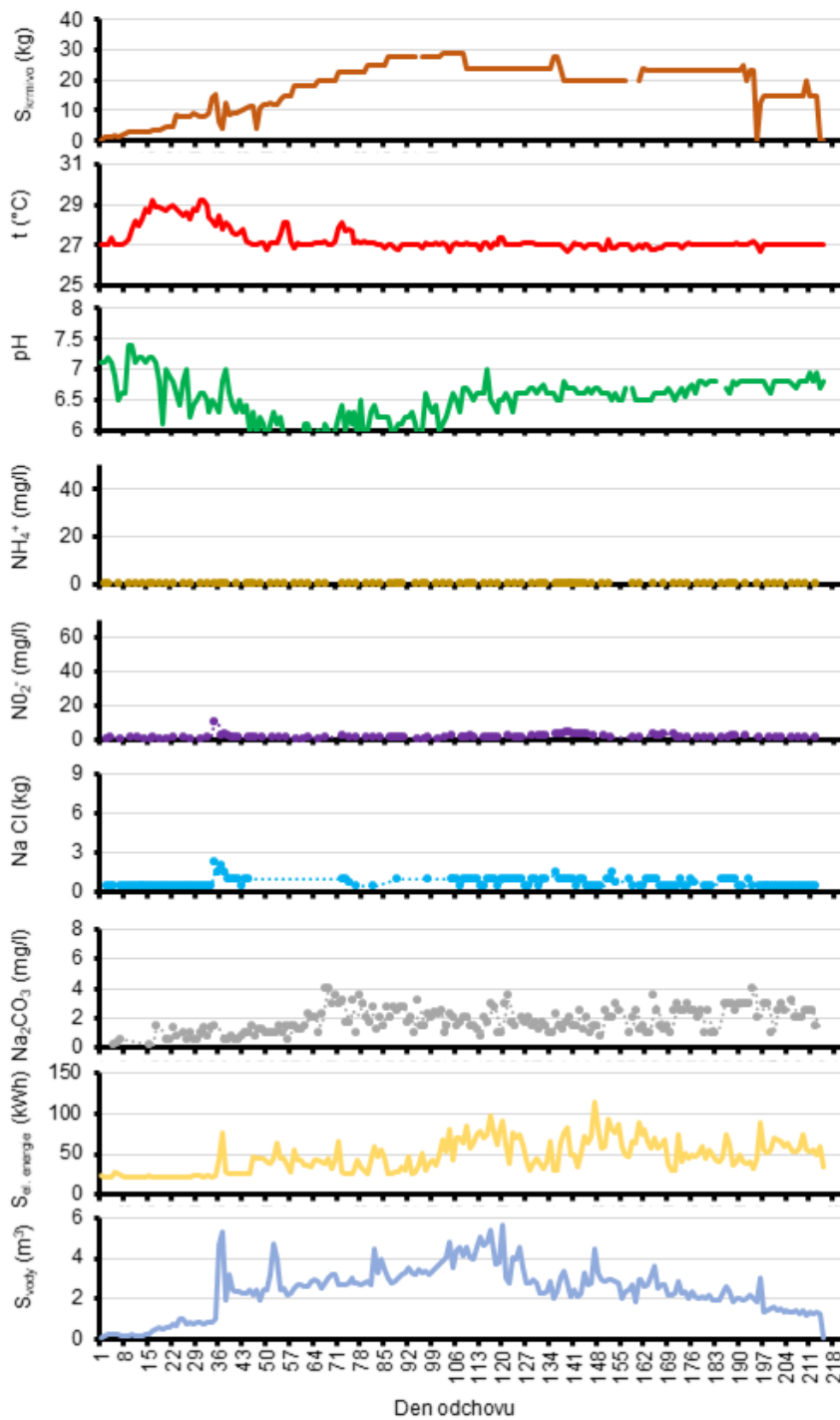
Graf 7. Aplikace krmiva, průběh fyzikálně chemických parametrů vody, spotřeby soli, sody elektrické energie a vody při odchovu keříčkovce červenolemého v recirkulačním systému farmy kontejnerového typu během prvotního odchovu s využitím krmiva Aller Aqua (Bona Float).
