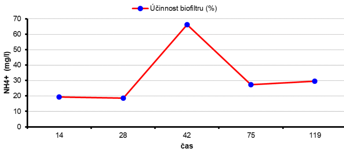
Graf 31. Vývoj účinnosti biofiltru (%) během druhého experimentálního odchovu keříčkovců červenolemých odchovávaných pomocí krmiva Skretting (Presta a Meerval) v recirkulačním systému farmy kontejnerového typu.
