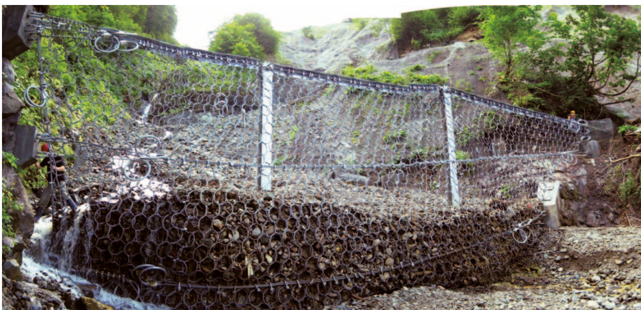
Obrázek 4-68: Ukázka zachycení splavenin pomocí dynamické bariéry UF 180 H6.
