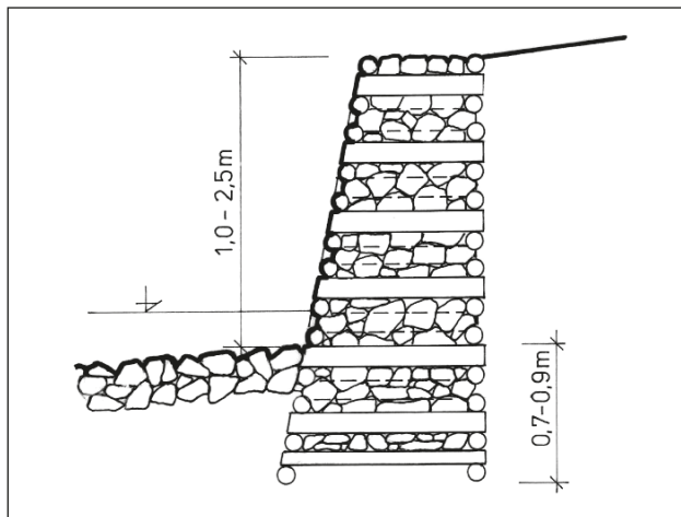
Obrázek 4-42: Dvoustěnná srubová stěna pro stabilizaci břehu, založená pod dno potoka. Zdroj: Zuna, Jaroslav: Stavby pro plnění funkcí lesa (2008).
