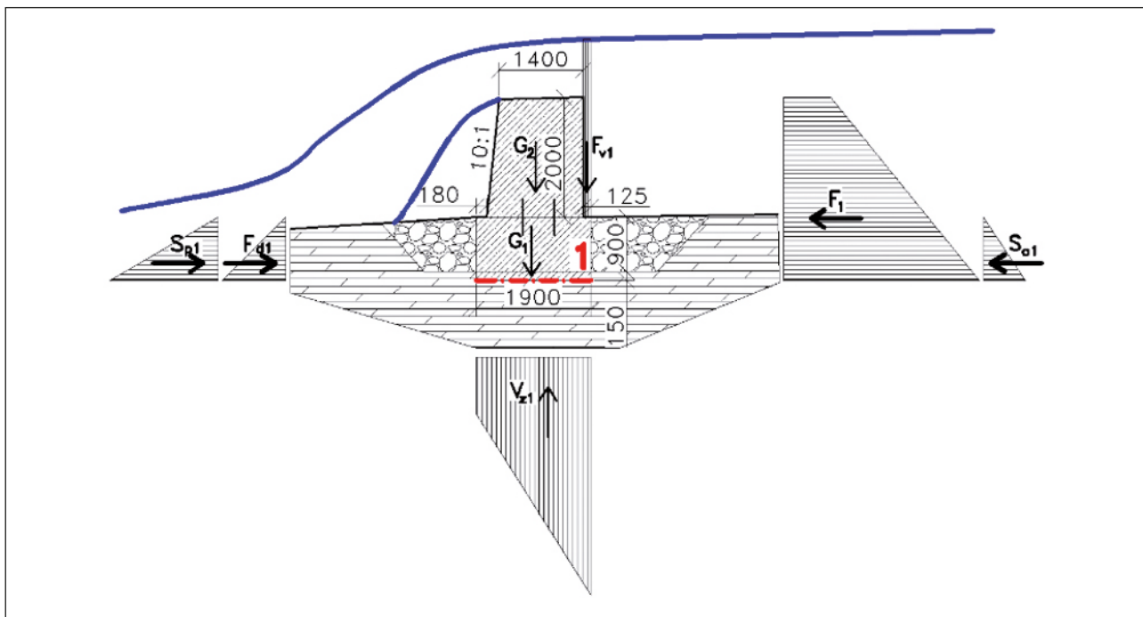
Obrázek 6-1: Posouzení v základové spáře č. 1.
