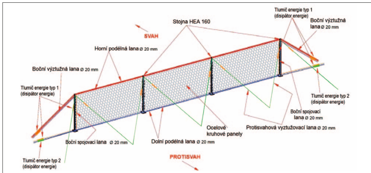
Obrázek 4-65: Flexibilní bariéra proti řízení skal – minimální garantovaná skladba polí. Autor: STRIX Chomutov, a. s.
