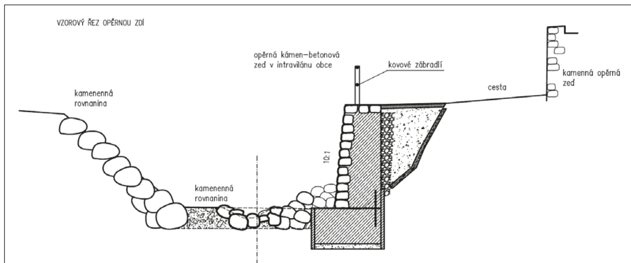
Obrázek 4-55: Ukázka možného řešení složeného profilu bystřiny v intravilánu s opěrnou zdí na pravém břehu a s rovinaninou z velkých kamenů na levém břehu.
