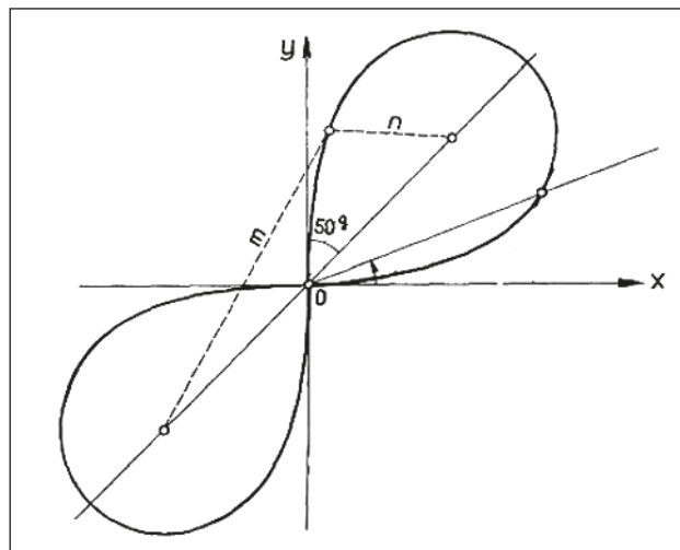
Obrázek 7-1: Bernoulliho křivka.
