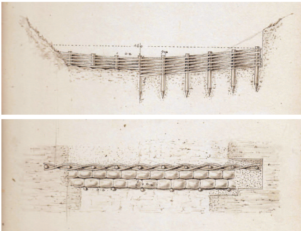
Obrázek 4-40: Boční a horní pohled na vrbový plůtek pro zpevnění svahů nad korytem – alternativu k latovým plůtkům. Skenováno z projektové dokumentace pro úpravu Okrouhlického potoka (zdroj: Lesy České republiky, s. p. – Odbor vodního hospodářství, archiv).
