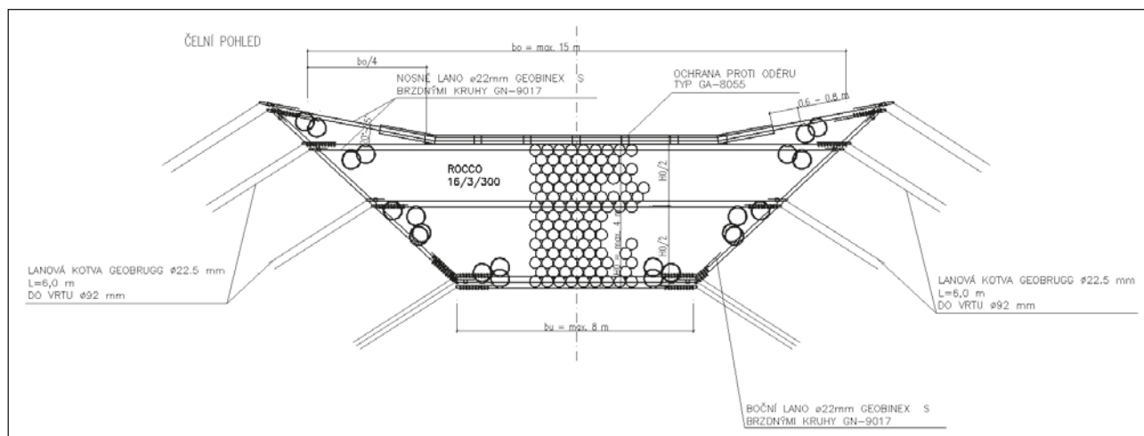
Obrázek 4-65: Flexibilní bariéra proti řízení skal – minimální garantovaná skladba polí. Autor: STRIX Chomutov, a. s.
