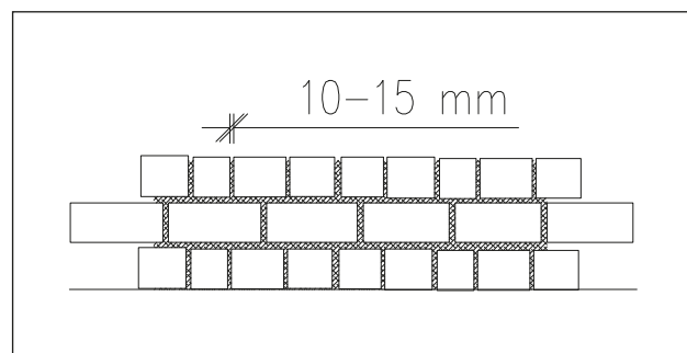
Obrázek 4-58: Čistě řádkové zdivo.
