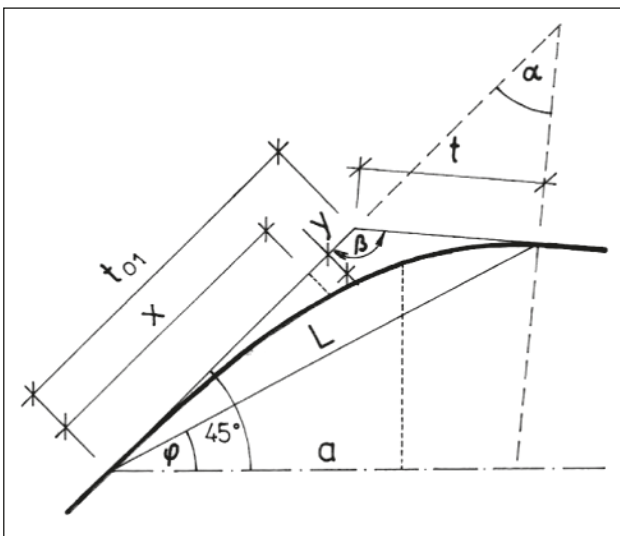
Obrázek 7-3: Nesouměrný lemniskátový oblouk.
