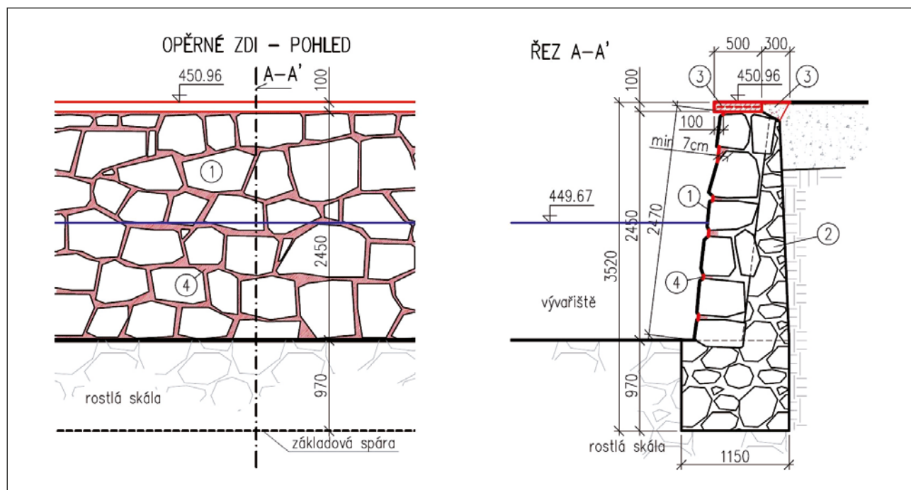
Obrázek 4-57: Ukázka režného kamenného zdiva.
