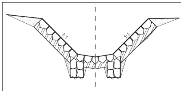
Obrázek 4-47: Kamenná dlažba do betonu ve dně a na březích. V patě svahu je patrná patka zděná z kamene. Dno je upraveno do středové střelky pro zajištění hloubky minimálních průtoků.
