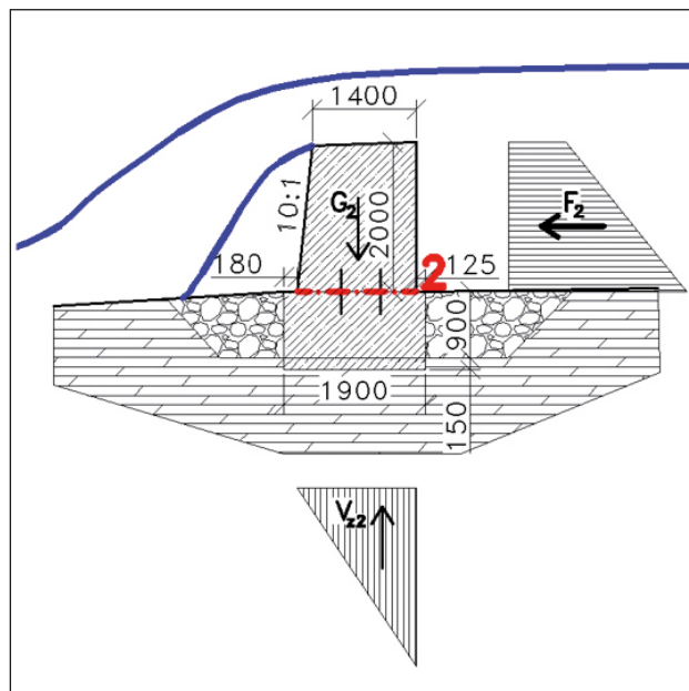
Obrázek 6-2: Posouzení v pracovní spáře č. 2.
