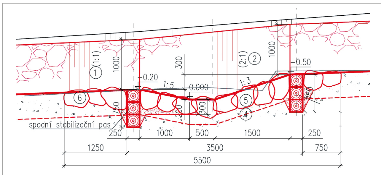
Obrázek 4-6: Práh s navazujícím tůňovým skluzem.
