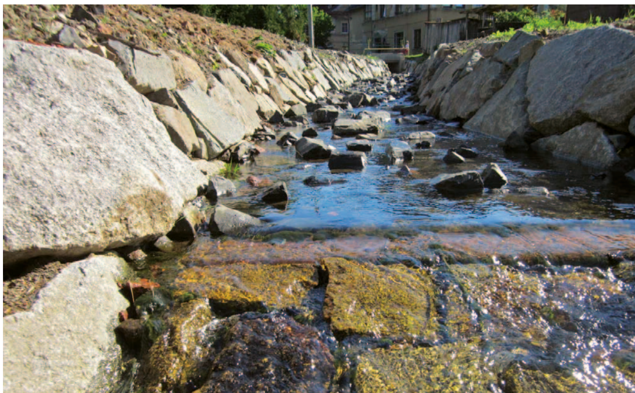
Obrázek 4-4: Pohled proti vodě na přechod dna koryta ve skluz, břeh je opevněn kamennou rovnaninou klínovanou kamenem. Opevnění dna v horní trati koryta je provedeno velmi hrubé z důvodu snížení energie vody, následně je sklonový přechod zpevněn dřevěným pasem z hraněné kulatiny, v březích je pas zatížen kamennou rovnaninou. Stabilizace pasem ve dně je nutná z důvodu změny rychlosti proudění vody na přechodu sklonů (dalšími místy, kde se používá stabilizační pas, jsou místa přechodu jednoho typu opevnění v jiný).
