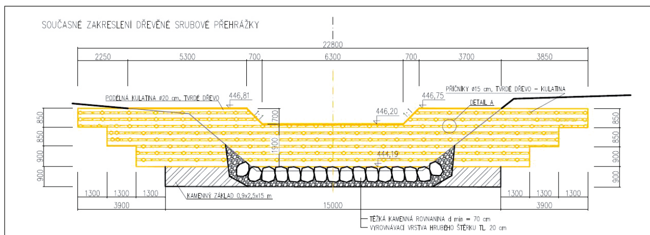
Obrázek 4-37: Pohled na konstrukci srubové přehrázky.
