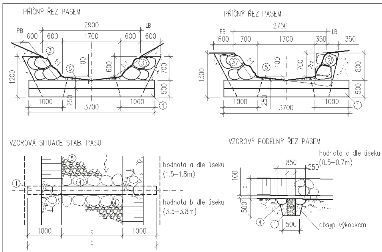
Obrázek 4-1: Dřevěný pas (na ložné hraně přitesaných kulatin doplněn o kamennou rovnatinu).
