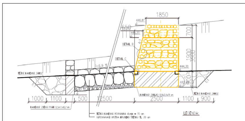
Obrázek 4-36: Řez srubovou přehrázkou se spadištěm ze štetovaného kamene.
