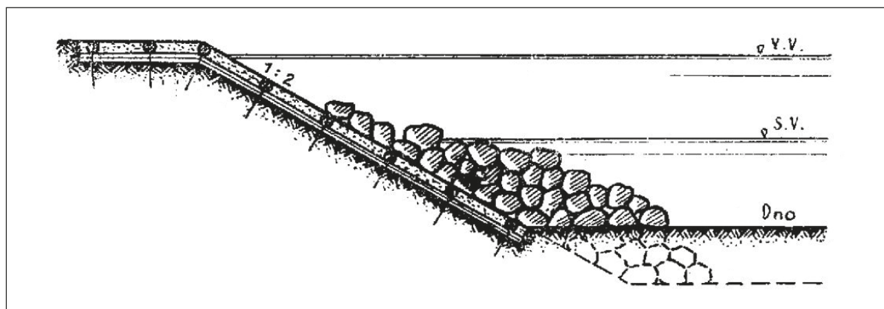
Obrázek 4-70: Zpevnění břehu vrbovou krytinou a paty svahu kamenným záhozem. Zdroj: Hlavinka, Vincenc: Nauka o melioracích, úpravách toků a hrazení bystřin – II. díl: Úprava toků a hrazení bystřin (1927).
